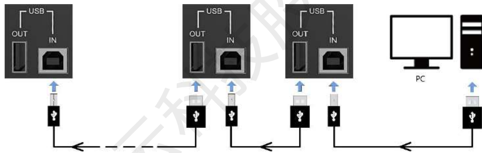
图4-1 设备级联示意图
